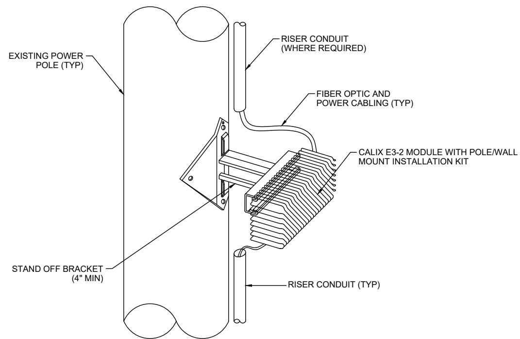
POLE MOUNT MODULE
