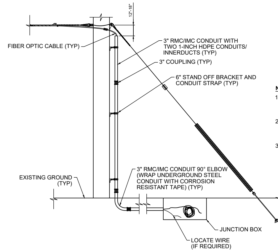
RISER CONDUIT DETAIL
