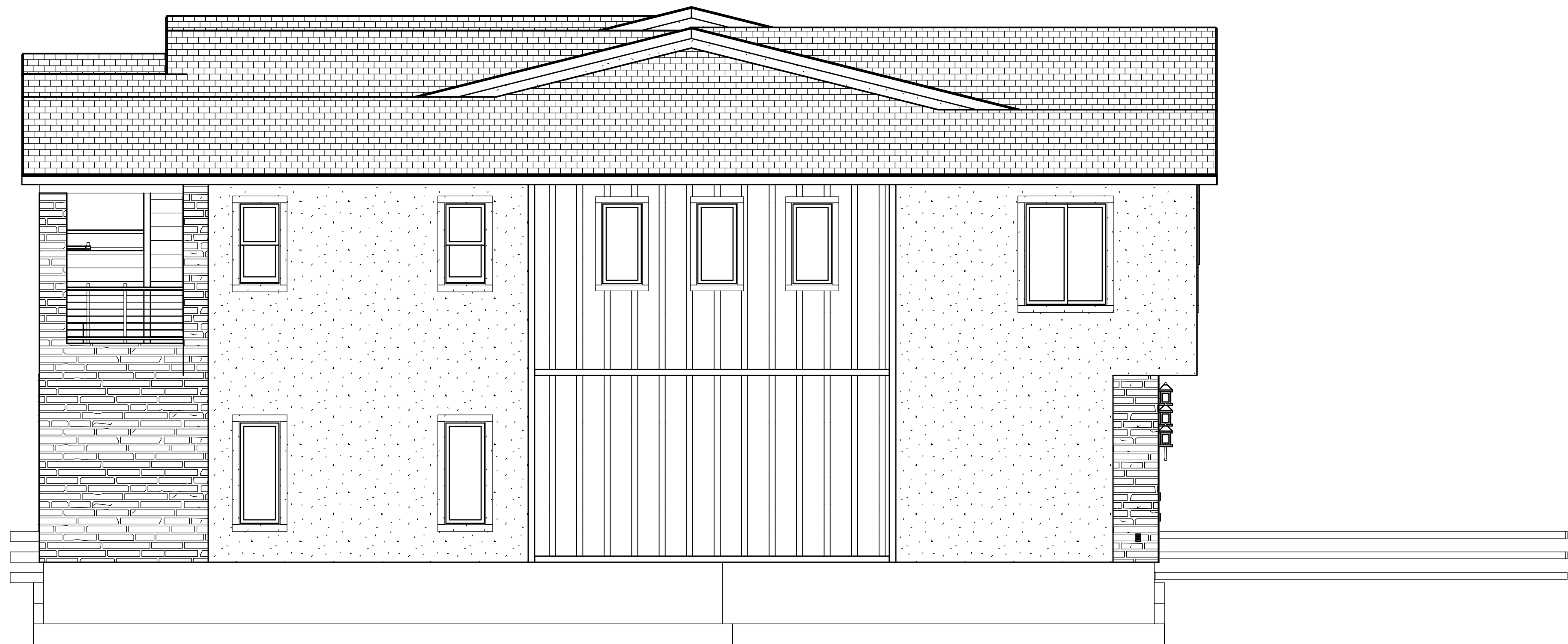
RIGHT ELEVATION
