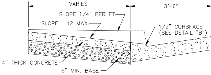
SECTION A-A
