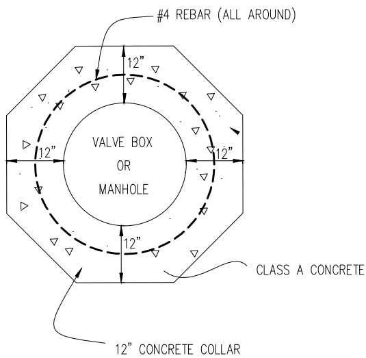
PLAN OPTIONAL
