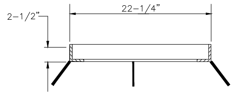
SECTION D-D
