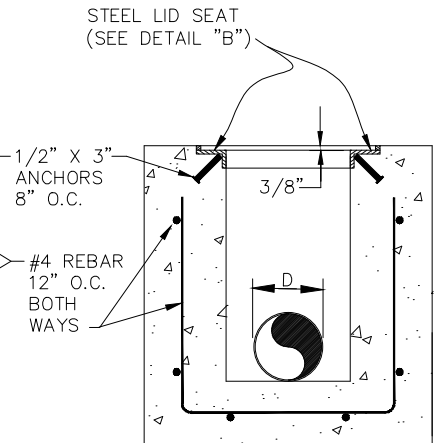
SECTION D-D
