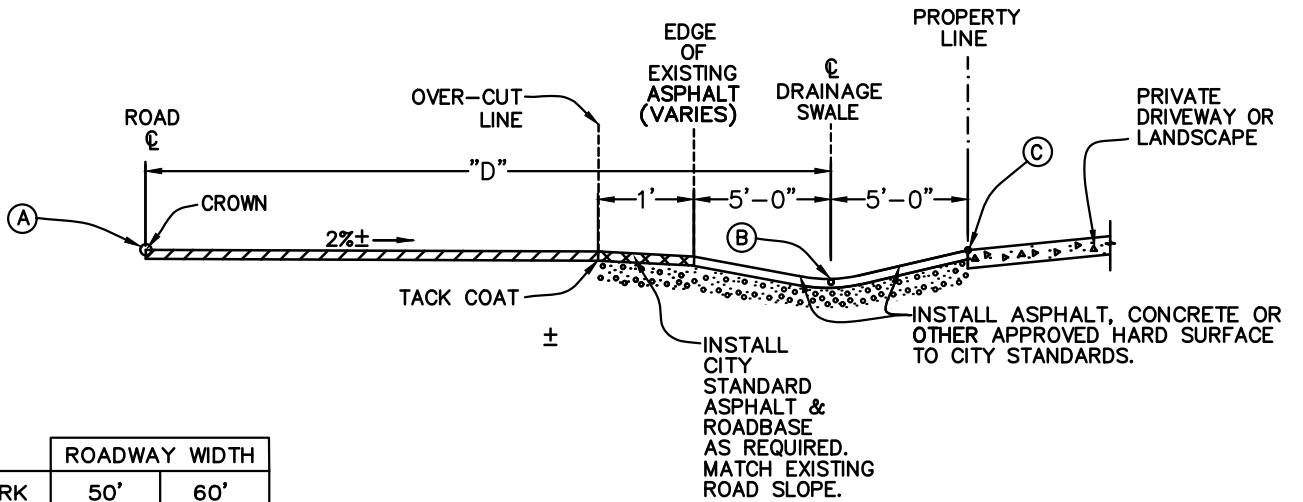
SECTION-A
