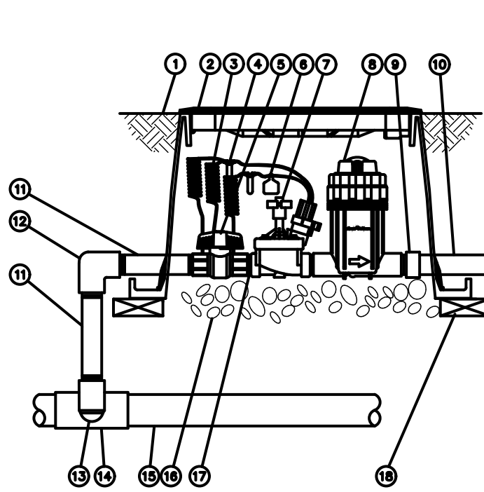
E DRIP VALVE ASSEMBLY N.T.S.
