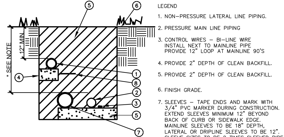
F PIPE-TRENCH-DETAILS SCALE: N.T.S.
