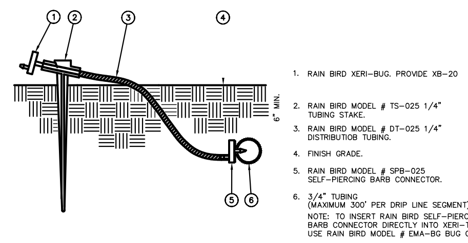
G EMITTER ASSEMBLY N.T.S.
