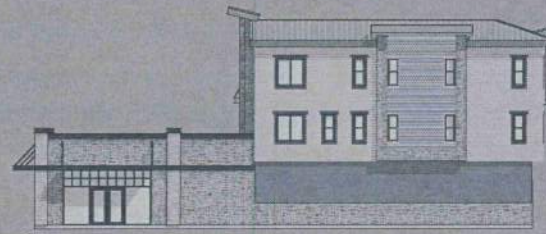
4 RIGHT ELEVATION SCALE: 1/8" = 1'-0"
