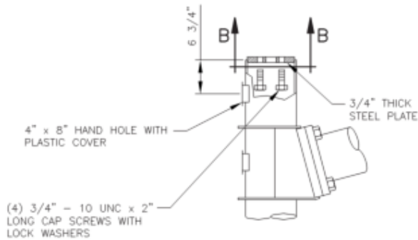
A3 BOTTOM CONNECTION SCALE: NTS
