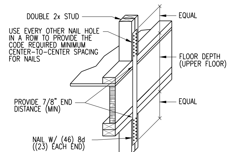
4 TYP. SIMPSON CS16 STRAP N.T.S.
