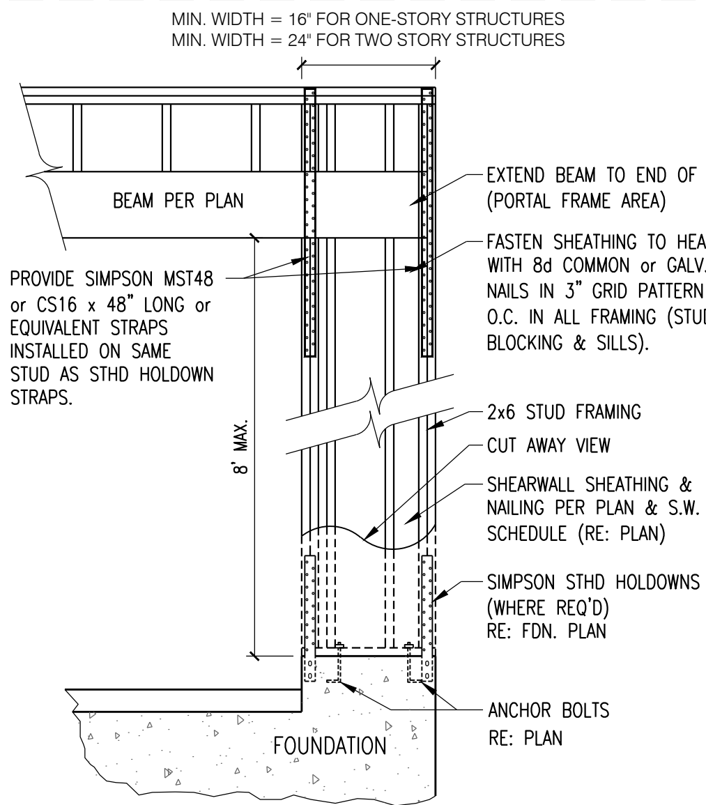
1 GARAGE RETURN DETAIL N.T.S.
