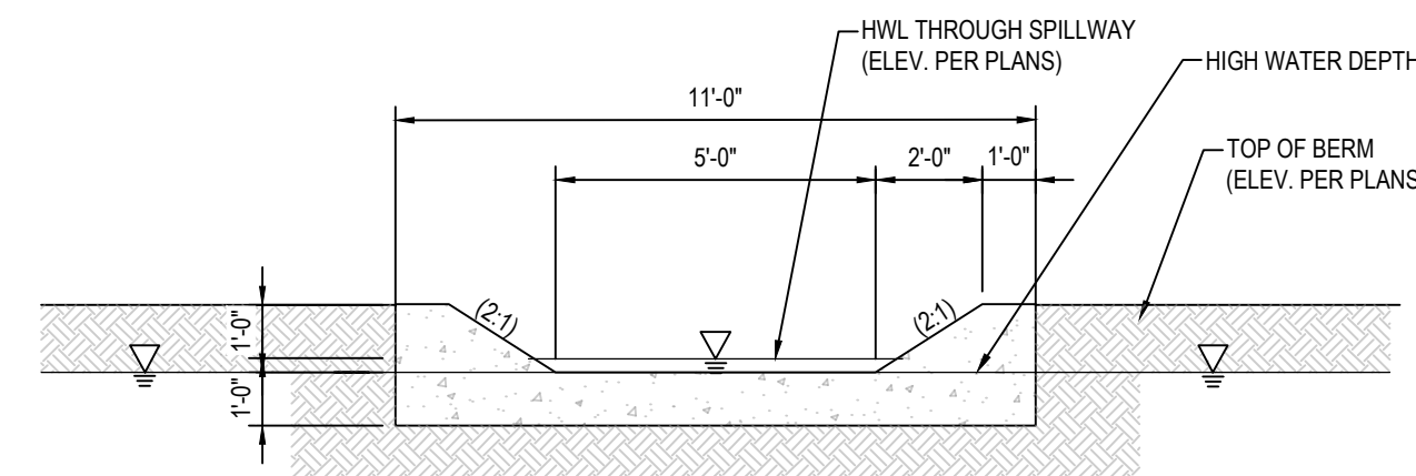
SECTION A-A
